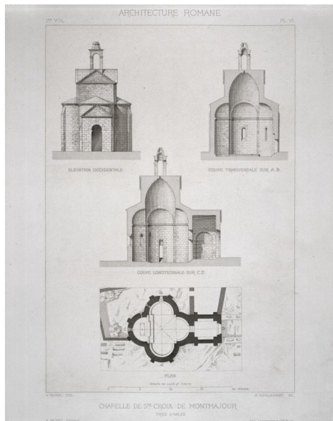
06. Plan de la chapelle Sainte-Croix © reproduction Philippe Berthé / CMN
